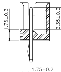
SEC. A-A
